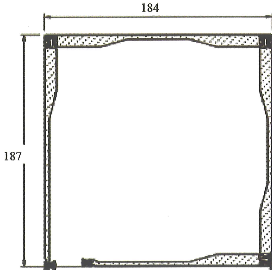
SECCION DEL CAJON DE ALUMINIO “LUXE BOX”
